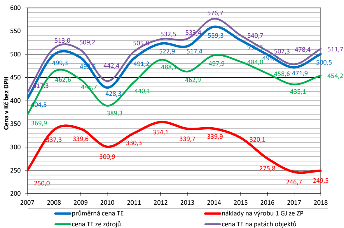
Vývoj - ceny tepelné energie a podílu proměnných nákladů (ZP) na výrobu 1 GJ
